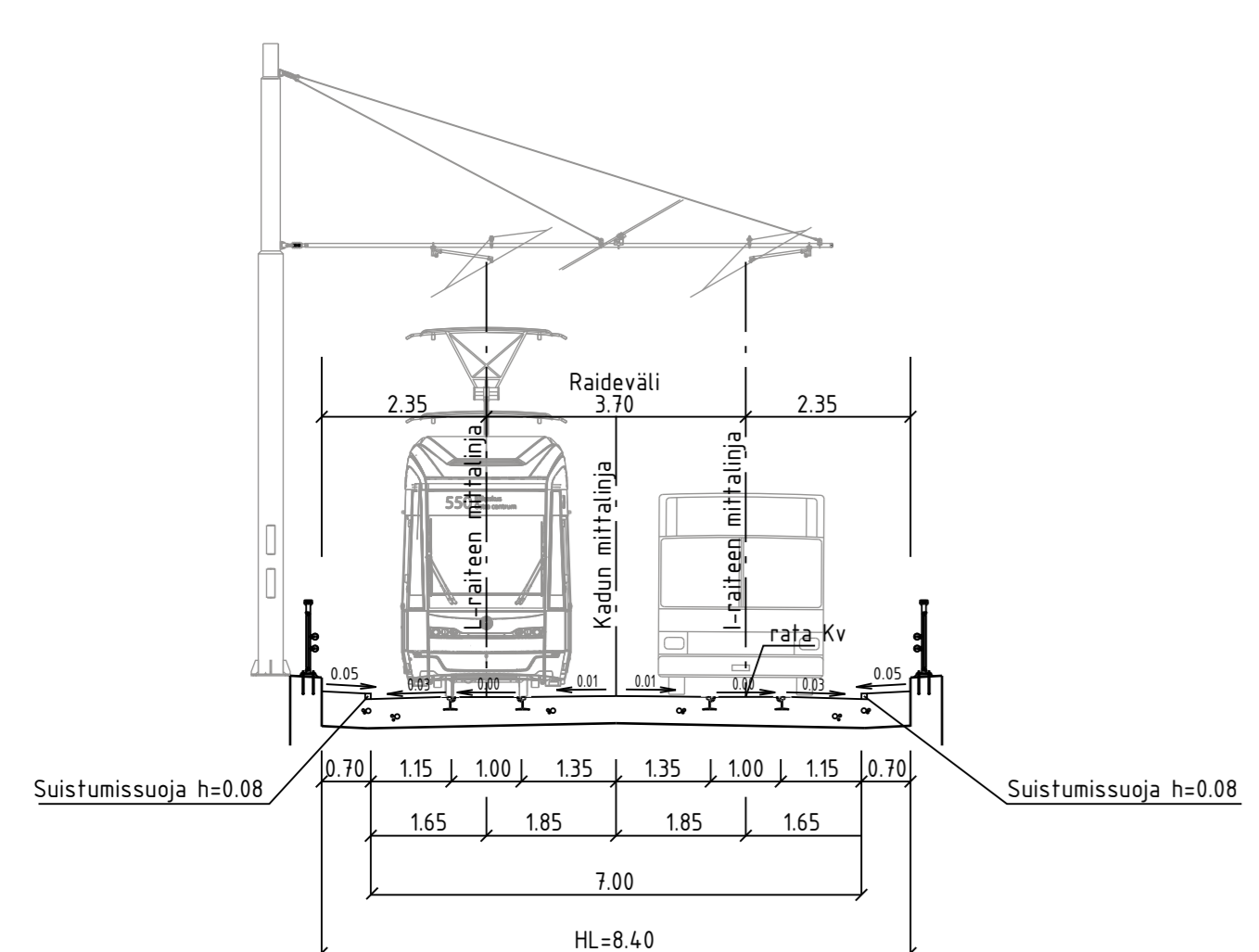
TYYPPIPOIKKILEIKKAUS A-A 1:100
